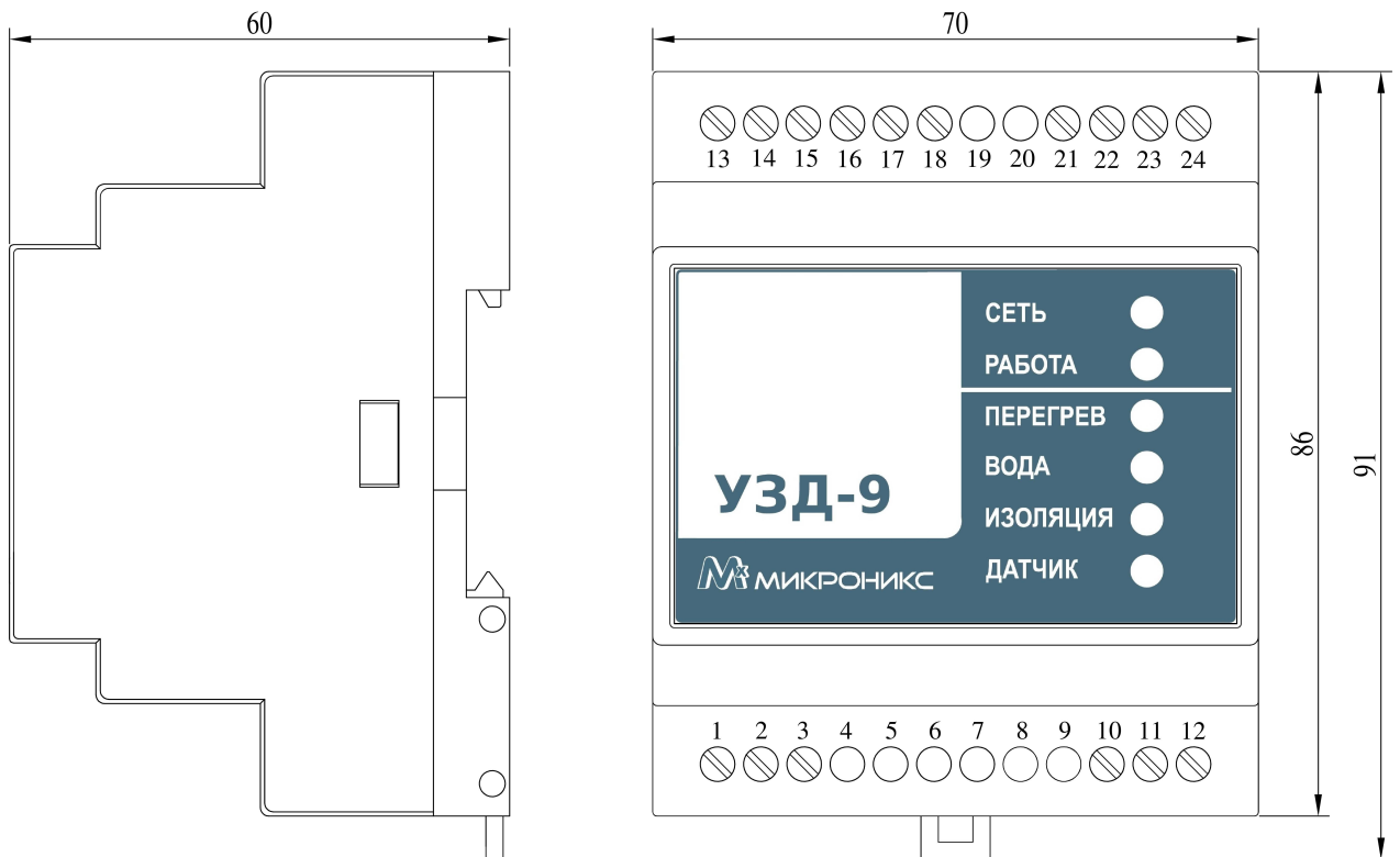
Рисунок 1б - Габаритные размеры изделия
