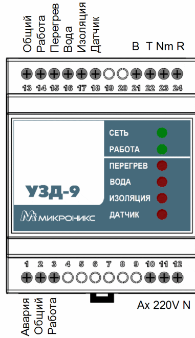
Рисунок 1а - Внешний вид устройства и назначение клемм
